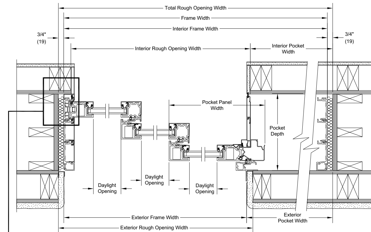
MMSD-PKT - XXXP
