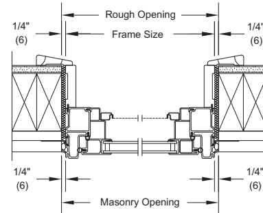
Jambs
