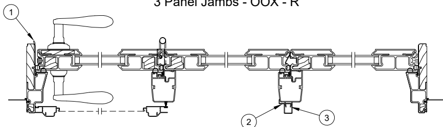
3 Panel Jamb - XOO - R
