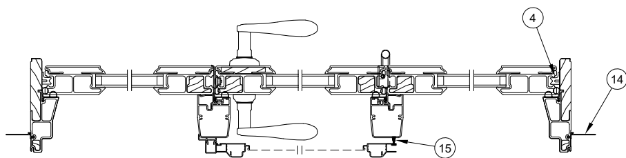
3 Panel Jamb - OXO - R
