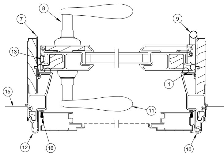
Jambs - X - R
