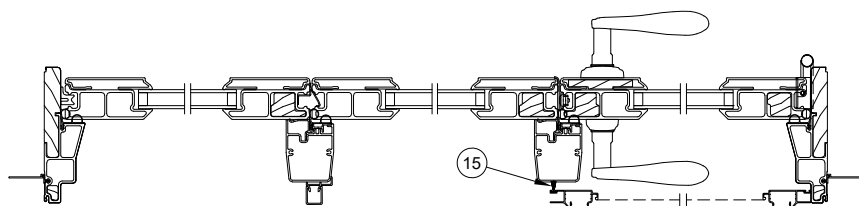
3 Panel Jamb - OOX - R
