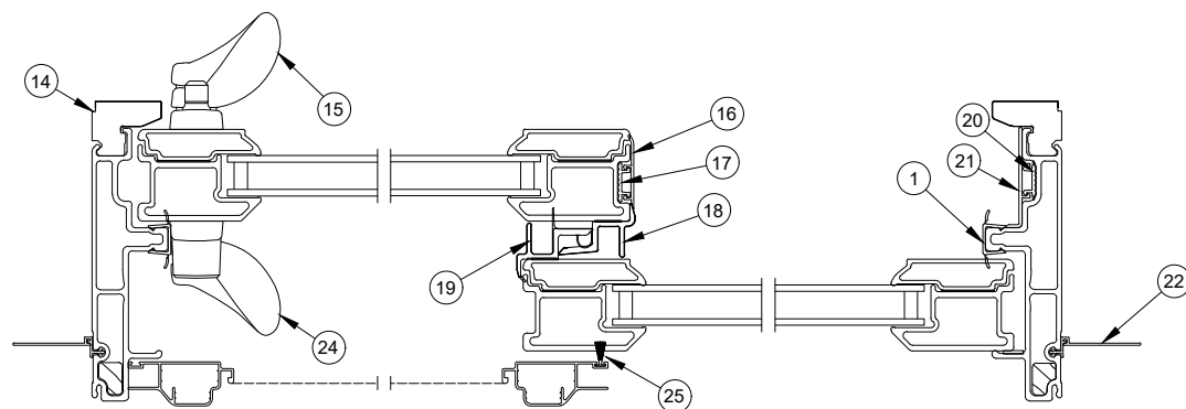
2-Panel XO - Jamb
