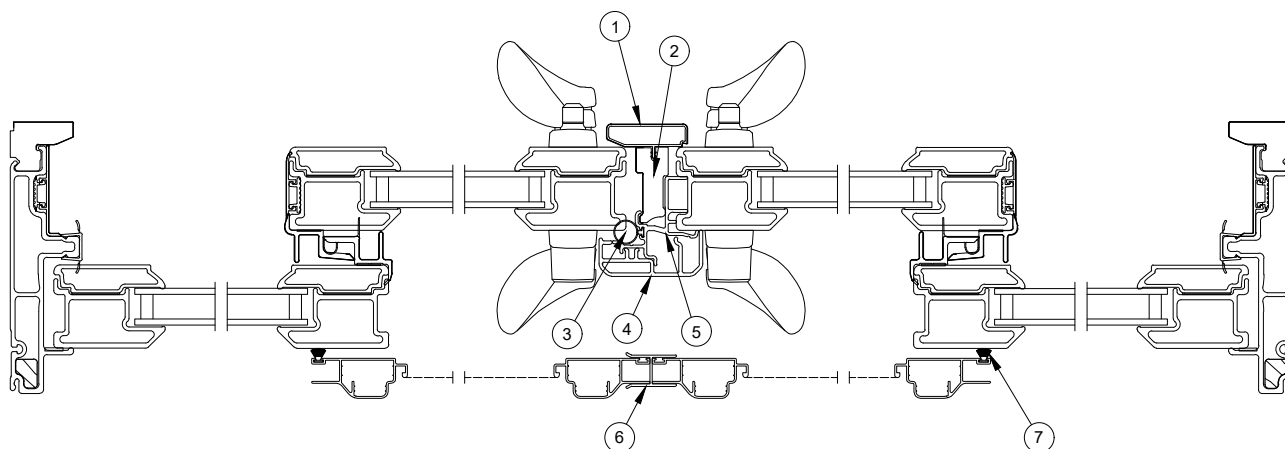
4-Panel Jamb Detail - OXXO
