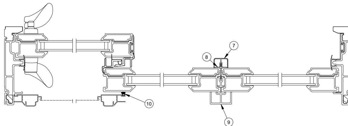
3-Panel Jamb Detail - XOO
