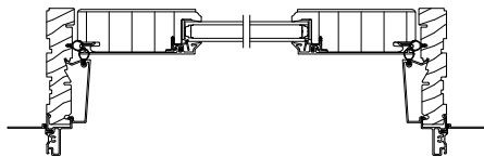
JAMB
