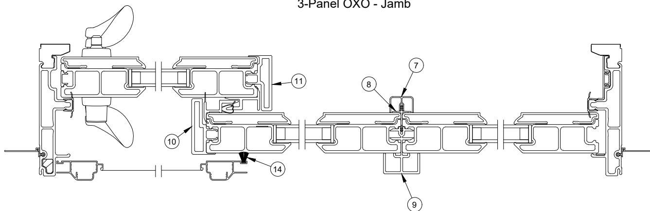
3-Panel XOO - Jamb
