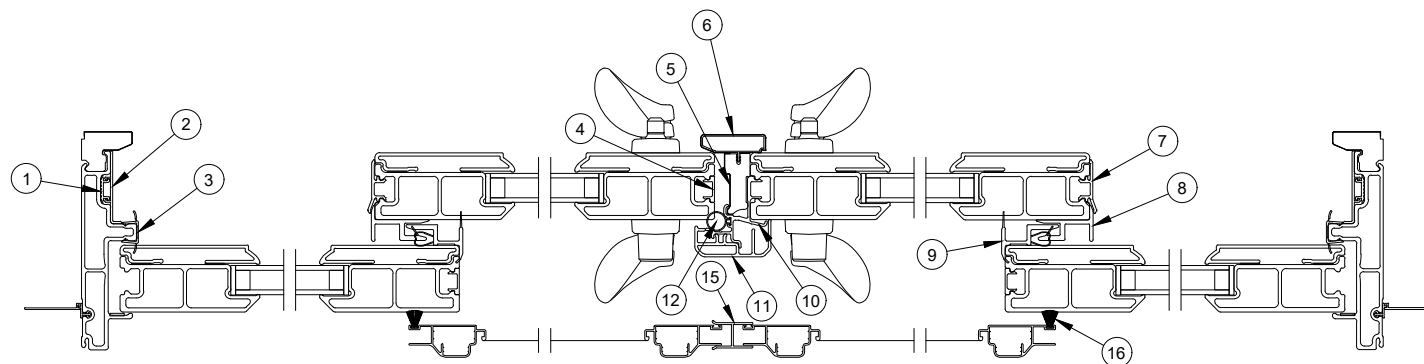
4-Panel OXXO - Jamb ≤86.00
