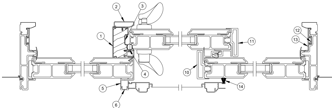
3-Panel OXO - Jamb
