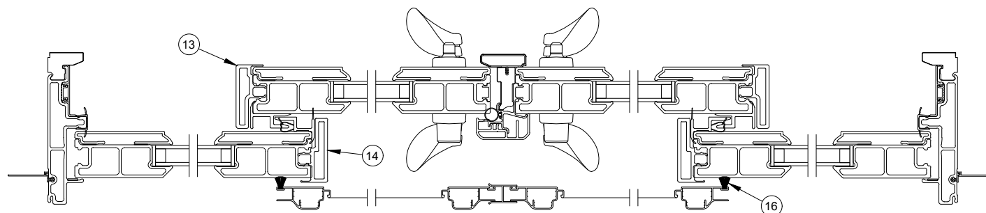
4-Panel OXXO - Jamb >86.00
