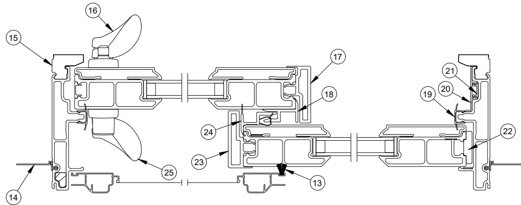
2-Panel XO - Jamb
