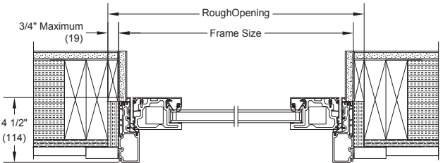
O JAMB
