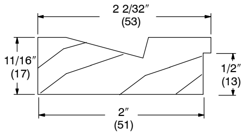
6 9/16" Jamb Extension, W7432
