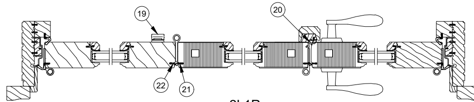
2L1R Jamb Details
