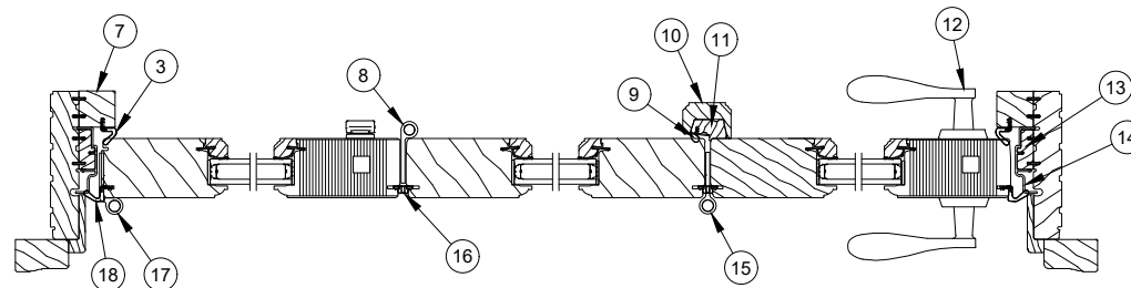
3L Jamb Details
