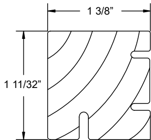
Jamb Part Stop, W12713
