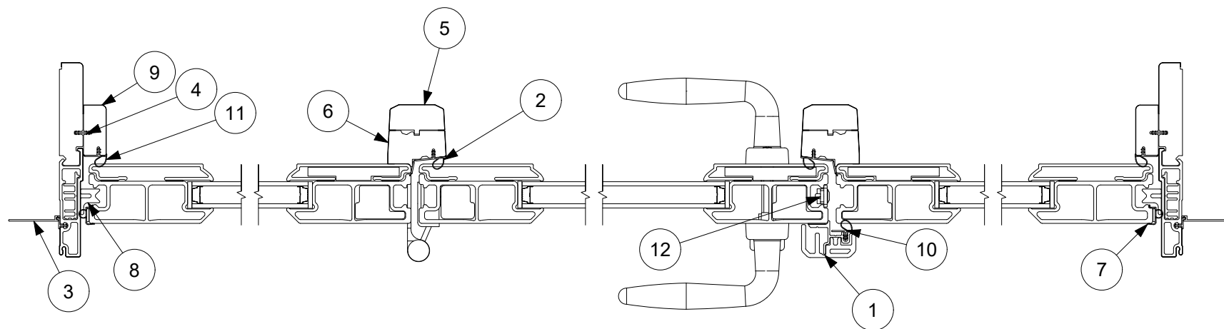
Jamb Detail
