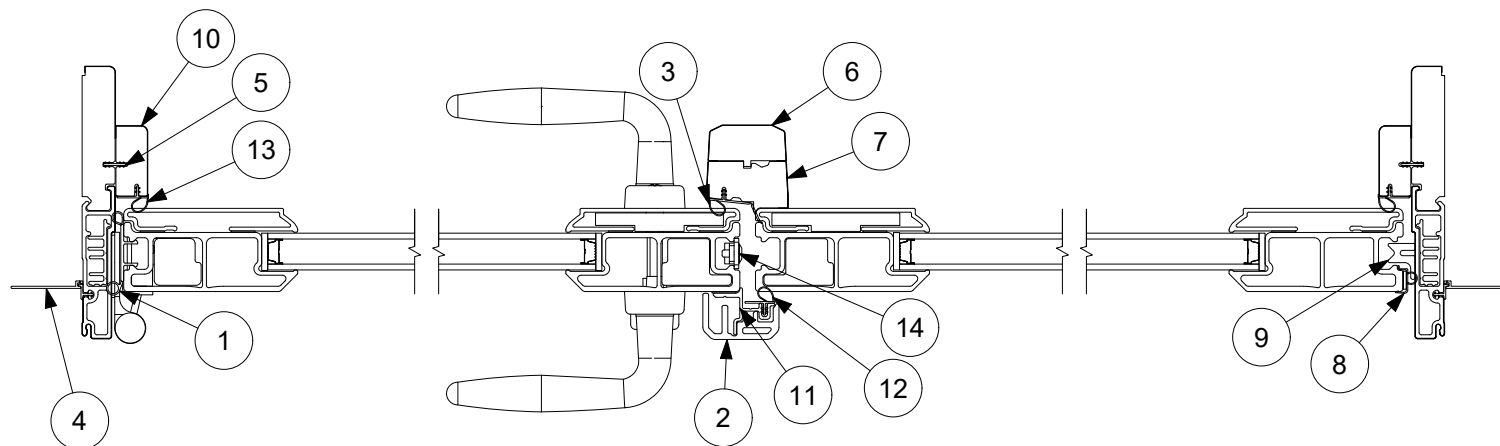
Jamb Detail
