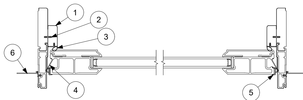
Jamb Detail
