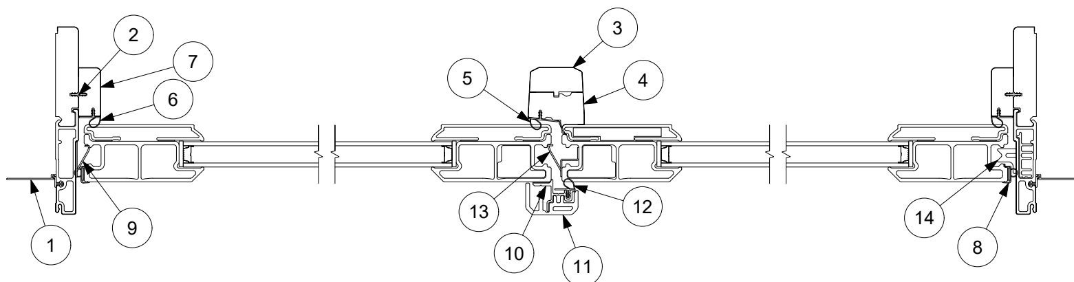
Jamb Detail
