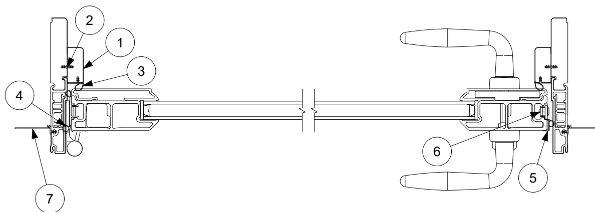
Jamb Detail
