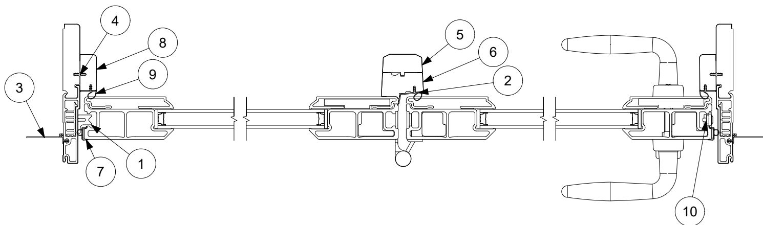
Jamb Detail
