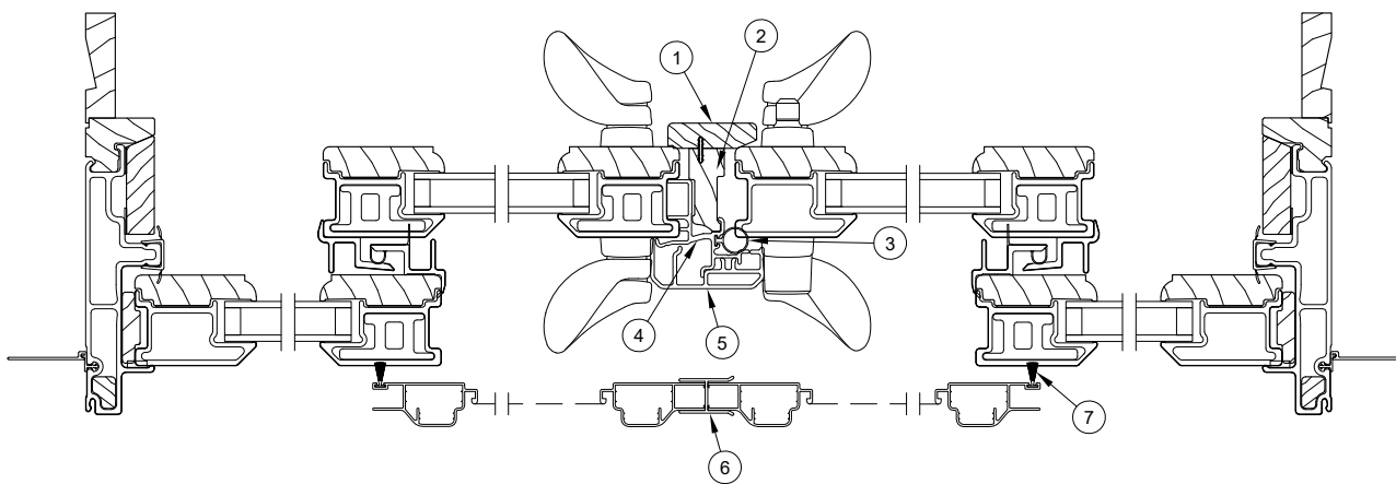
4 Panel Jamb Detail - OXXO R
