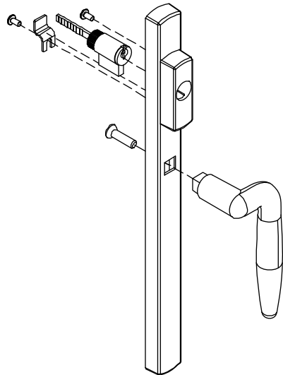
XO/OOX/OXO-R/OXXO-R shown
