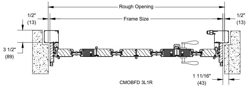
CMOBFD 3L1R
