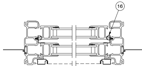
Jamb Detail
