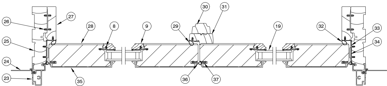
Jamb - Transom - OO (1 frame - 2 sash)
