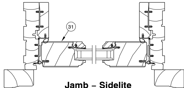
Jamb - Sidelite
