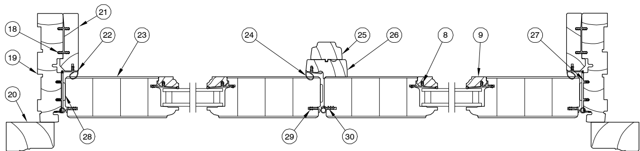
Jamb - OO
